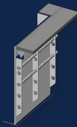
Typ 2 Overflow direkt über den Beckenrand
